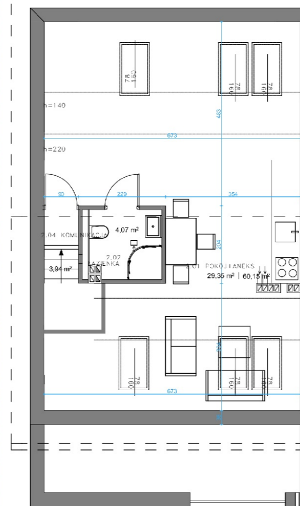
RZUT PODDASZA
