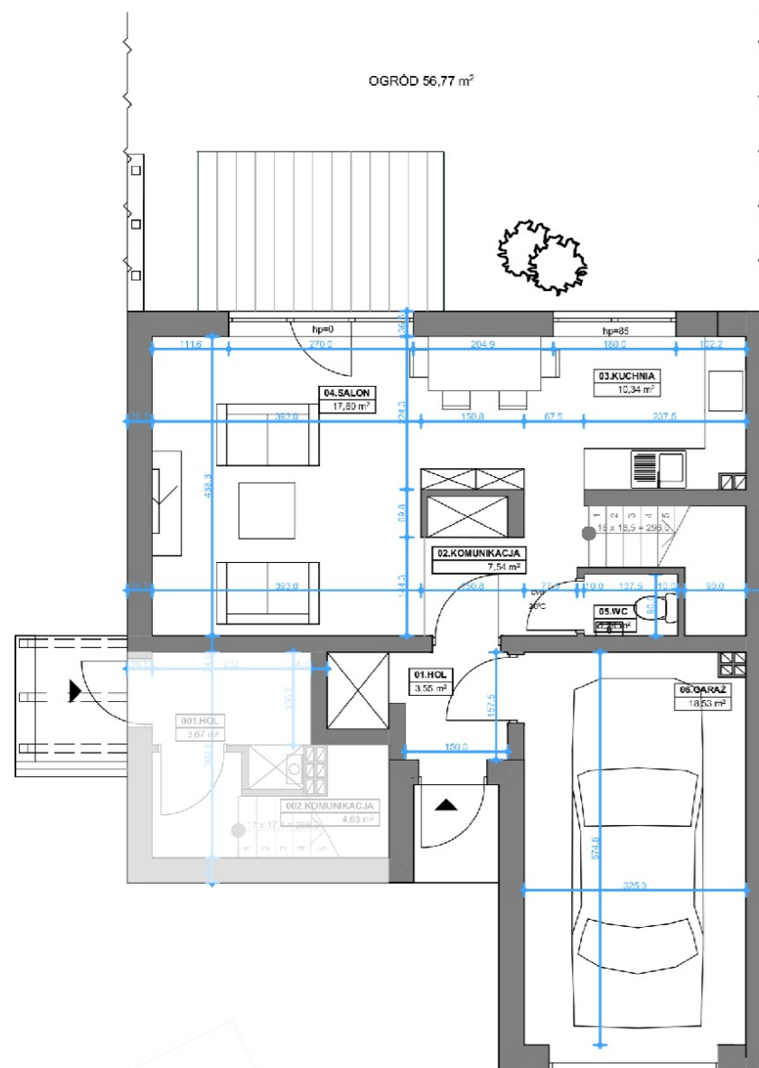
RZUT PARTERU
