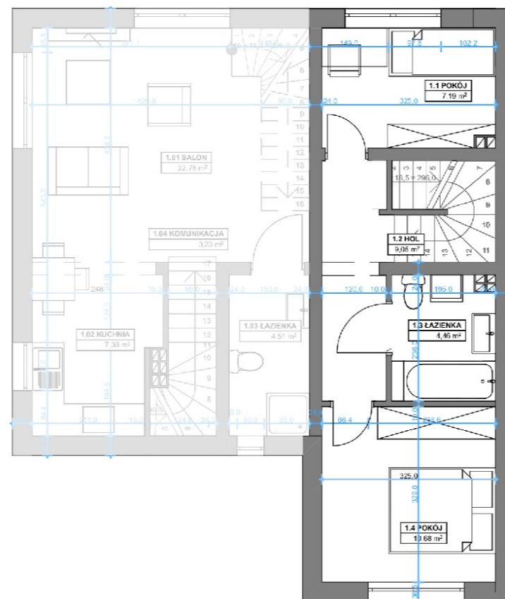
RZUT PIĘTRA
