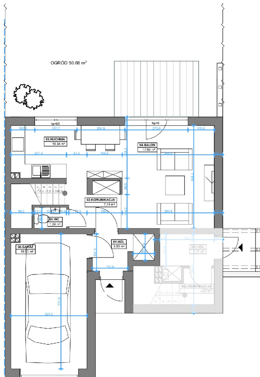
RZUT PARTERU
