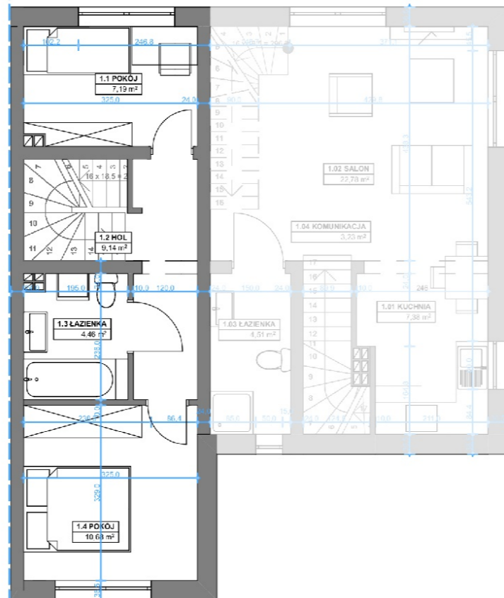
RZUT PIĘTRA
