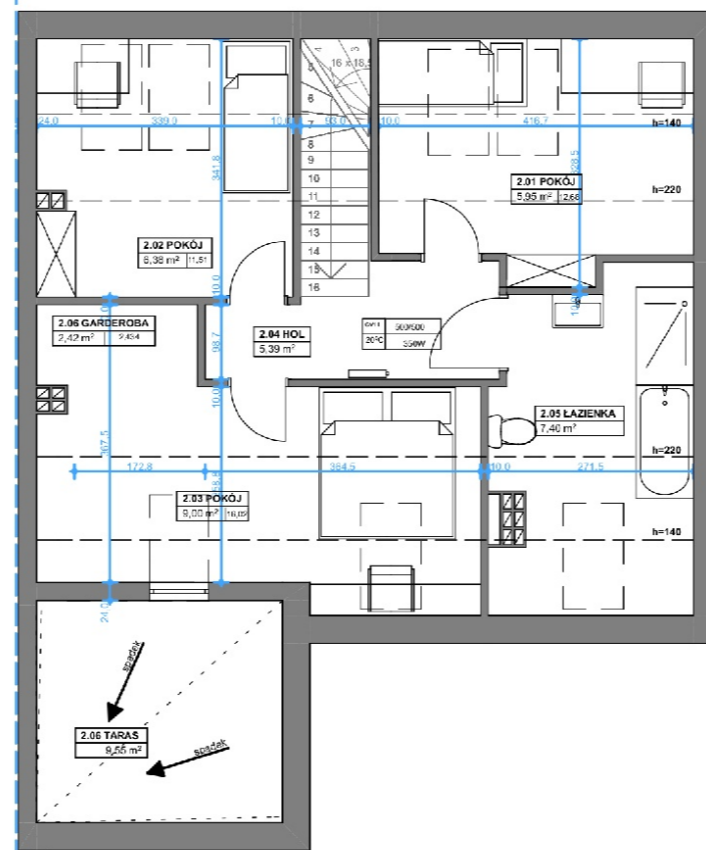
RZUT PODDASZA
