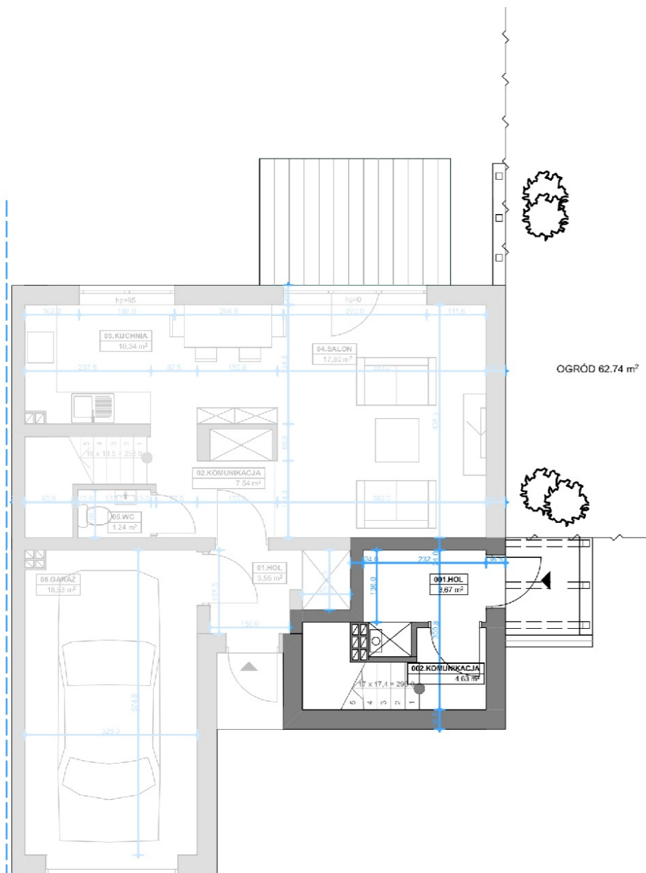
RZUT PARTERU
