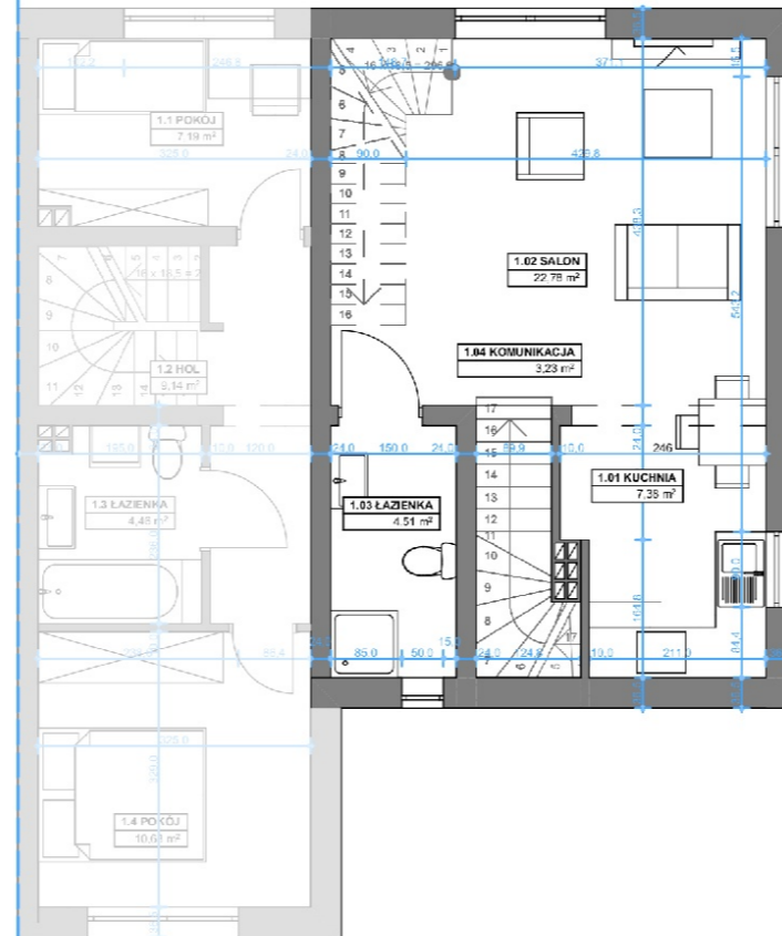
RZUT PIĘTRA
