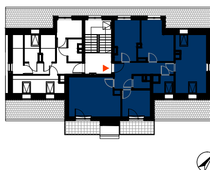
SCHEMAT KLATKI
