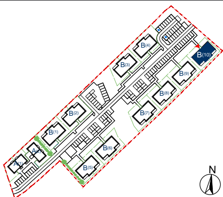
SCHEMAT ZESPOŁU
