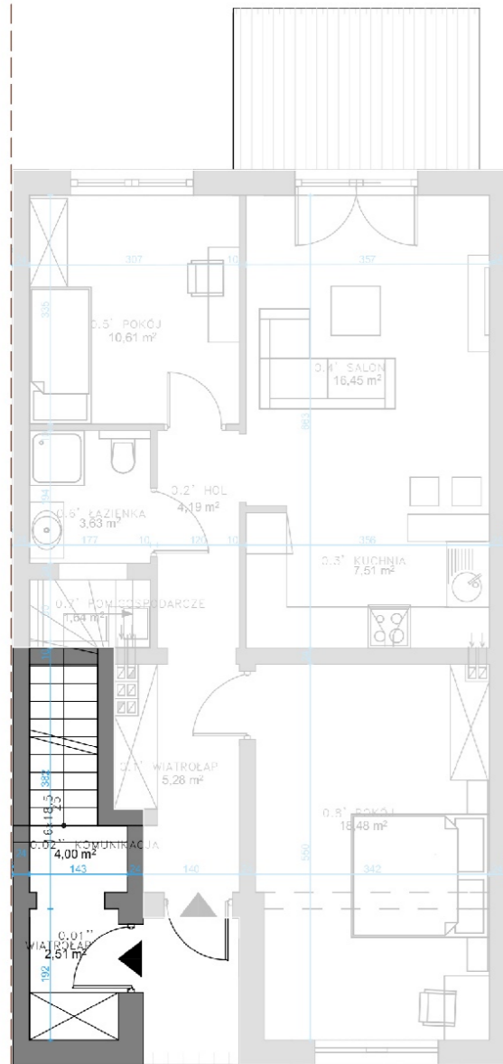
RZUT PARTERU
