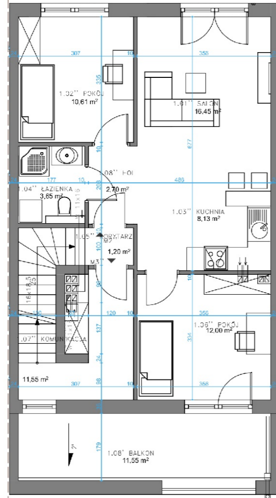
RZUT PIĘTRA
