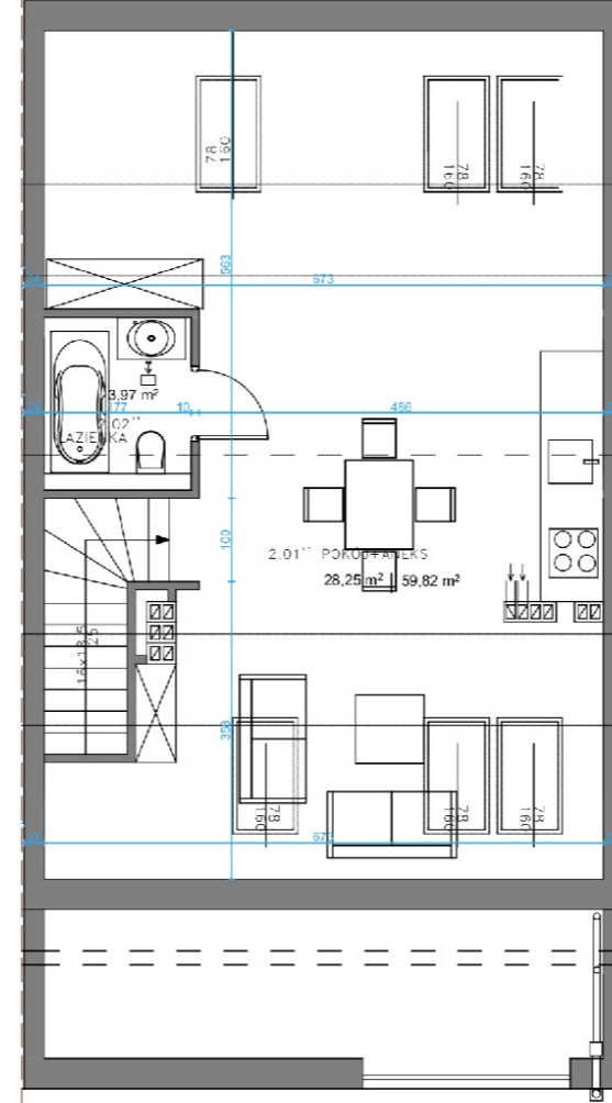
RZUT PODDASZA
