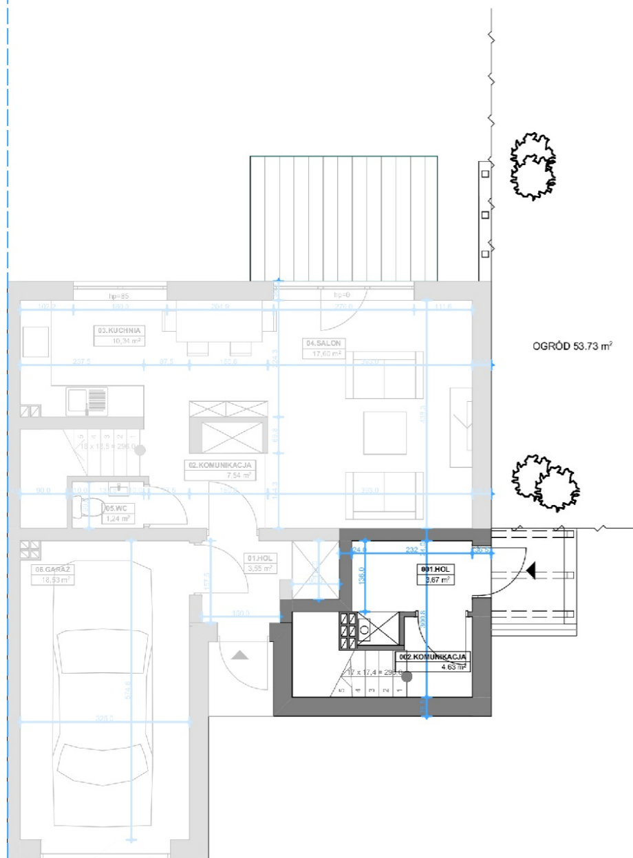
RZUT PARTERU
