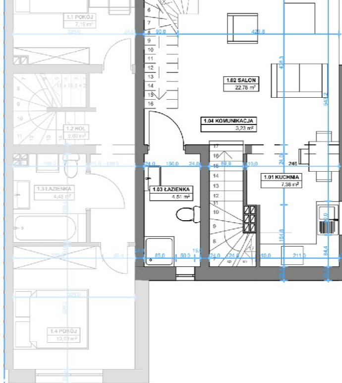
RZUT PIĘTRA
