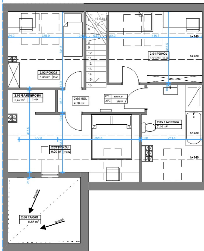
RZUT PODDASZA
