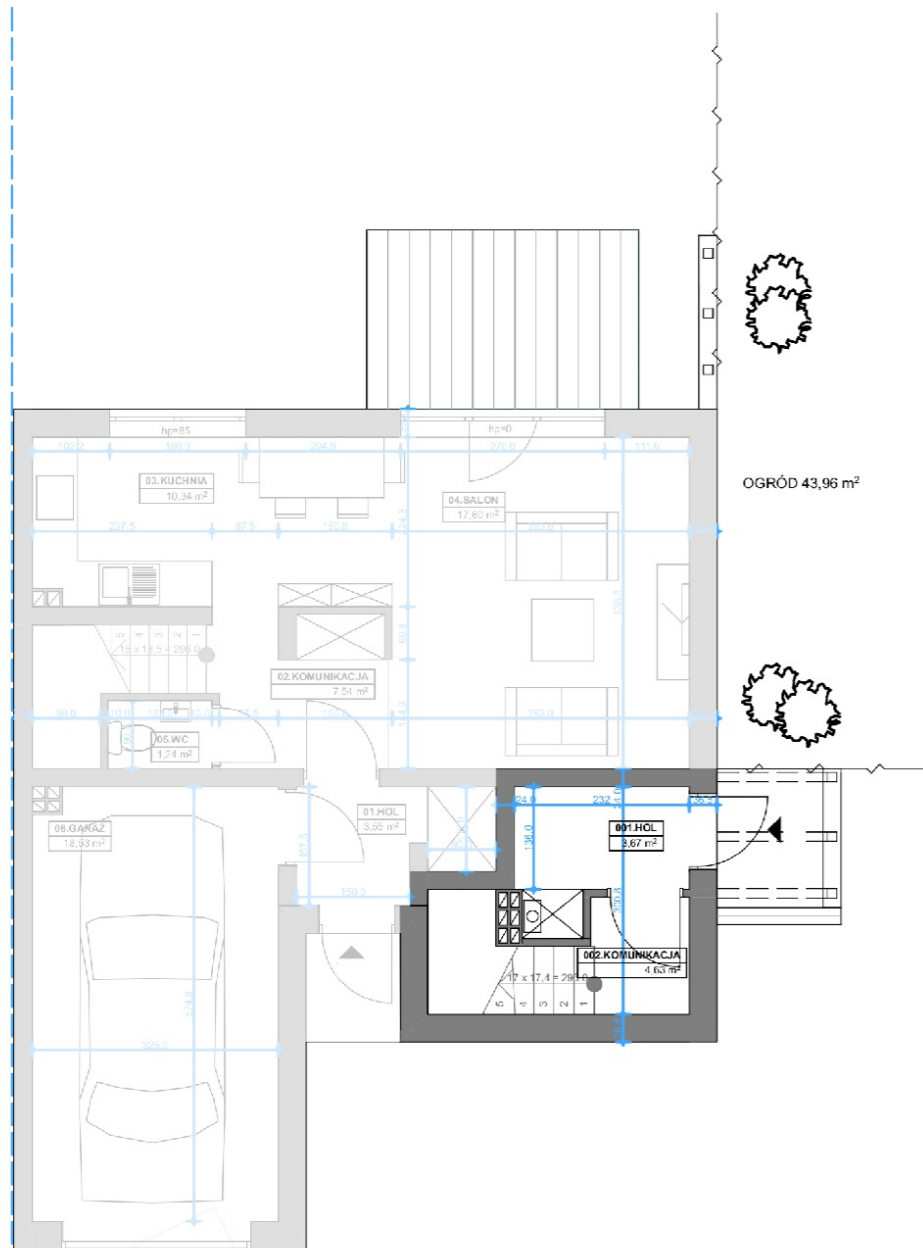
RZUT PARTERU
