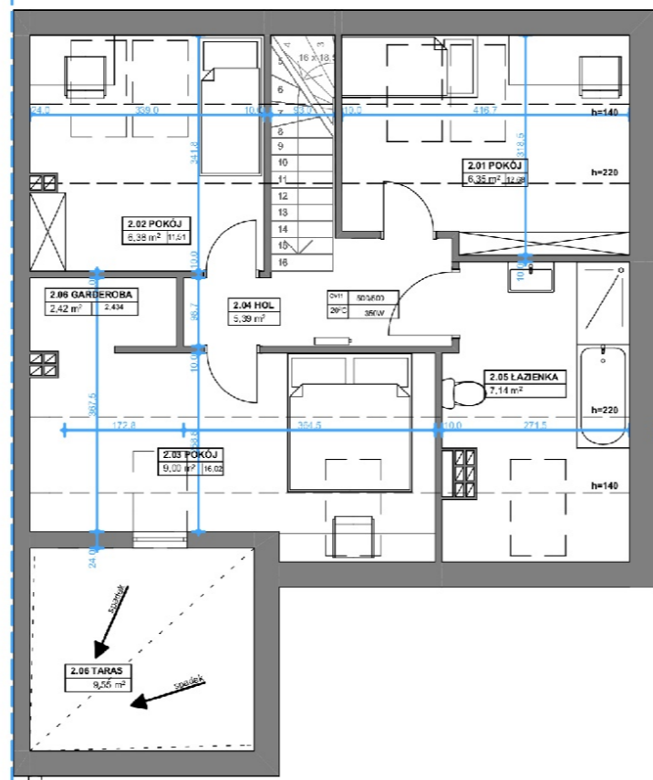
RZUT PODDASZA
