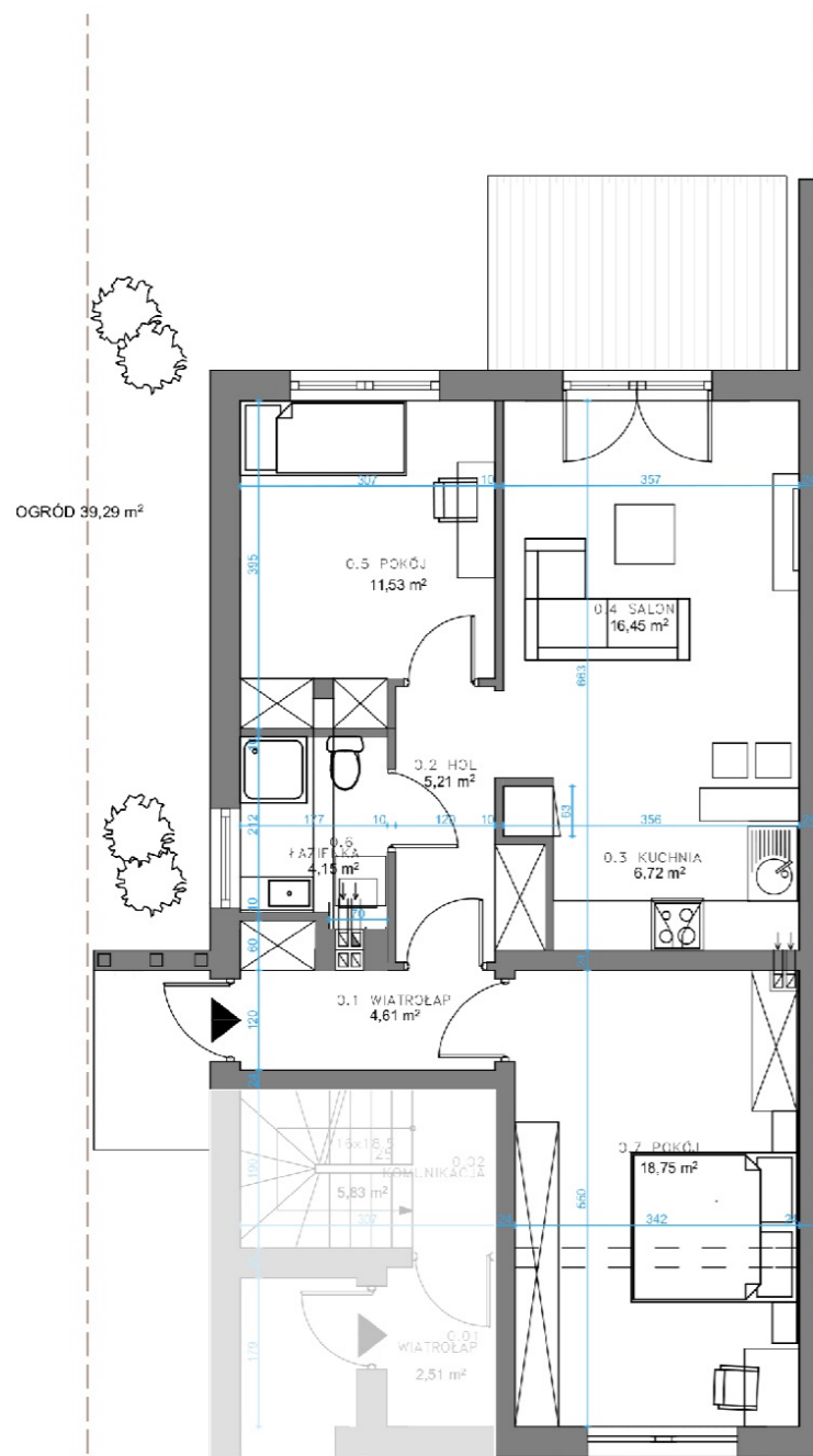
RZUT PARTERU
