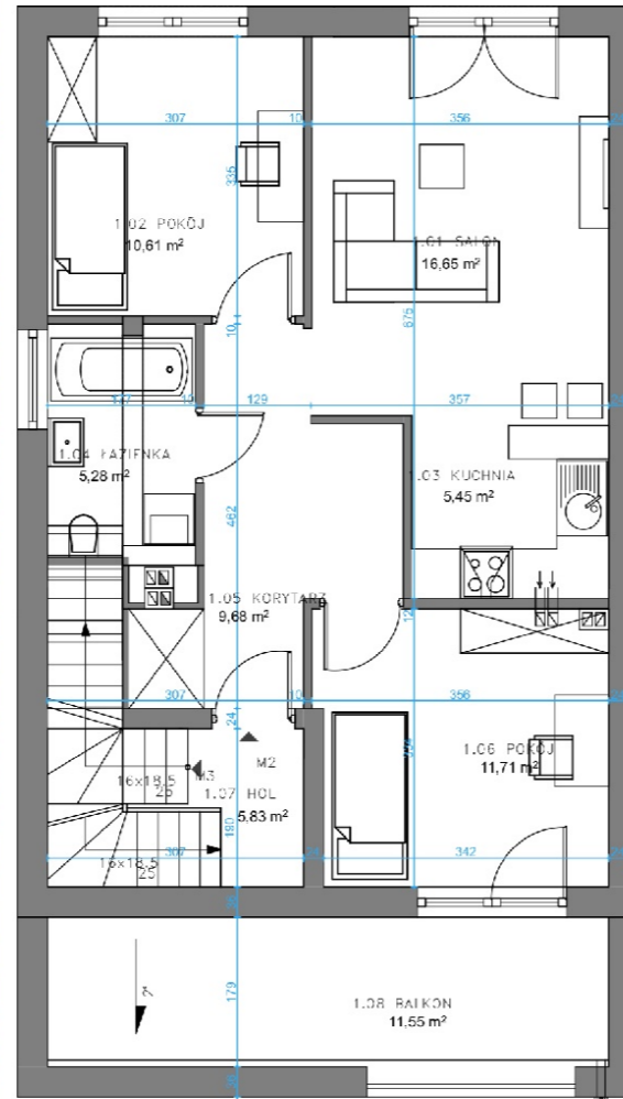
RZUT PIĘTRA
