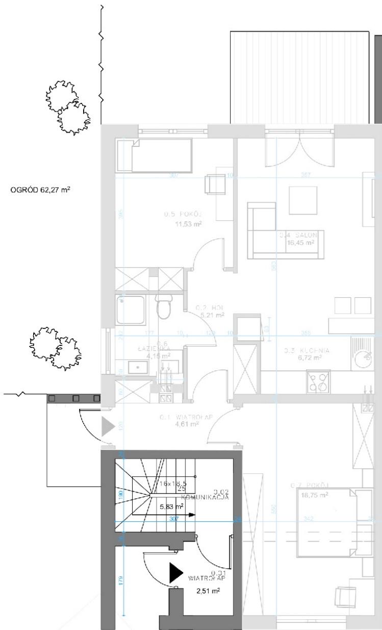
RZUT PARTERU
