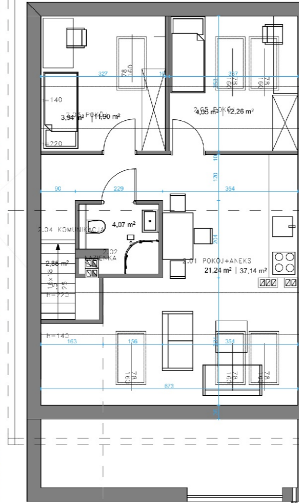
RZUT PODDASZA
