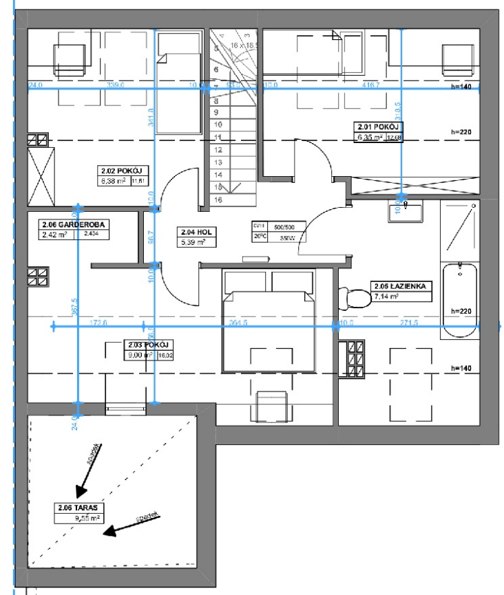
RZUT PODDASZA
