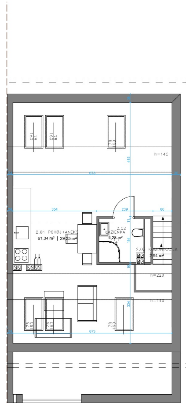
RZUT PODDASZA
