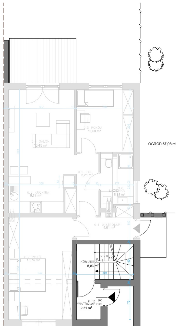
RZUT PARTERU
