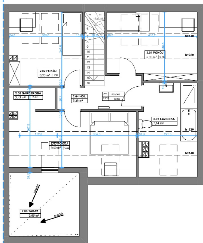
RZUT PODDASZA
