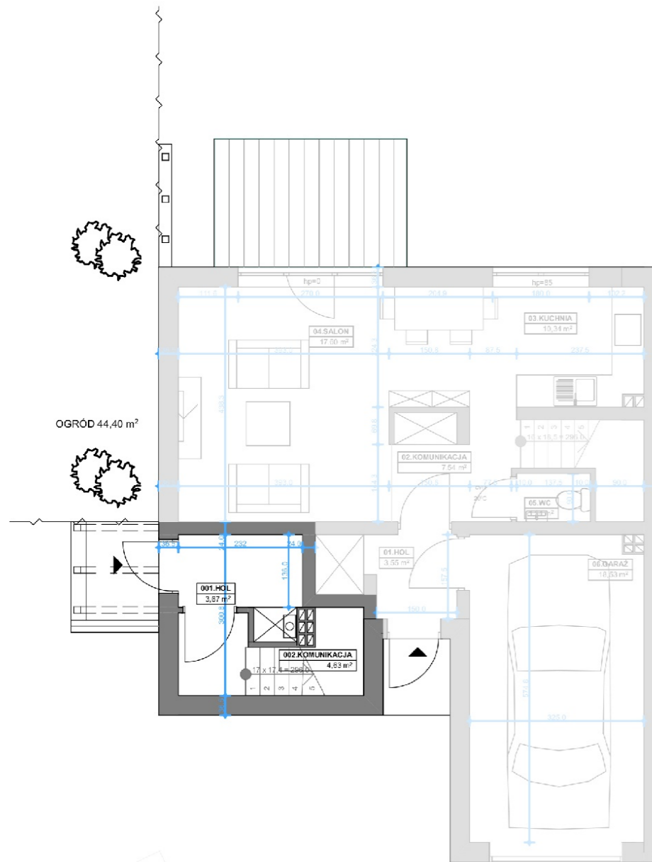
RZUT PARTERU
