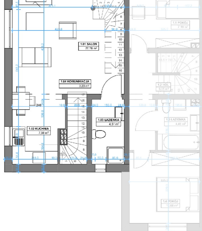
RZUT PIĘTRA
